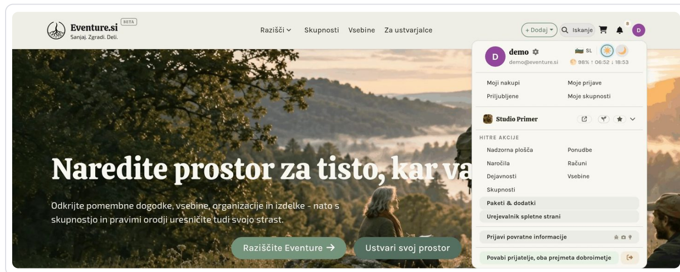
Posnetek zaslona 1.3. Meni z avtarjem: osebne postavke nad ločnico, vaša organizacija pod njo.
